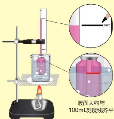
自制简易温度计 Homemade simple thermometer
