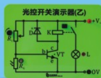
光控开关演示器(乙) Light Switch demonstrator (B)
