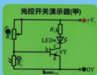
光控开关演示器(甲) Light Switch demonstrator (A)
