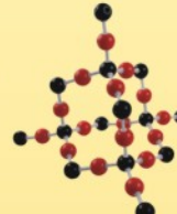
二氧化硅 (球棍模型) Silica (ball and stick model)
