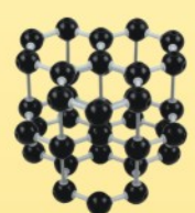
石墨分子模型 Graphite molecular model
