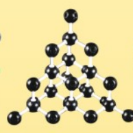
金刚石模型 Diamond model
