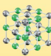
氯化钠晶体 Sodium chloride crystal
