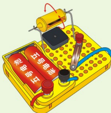
自制电动机 Homemade motor
