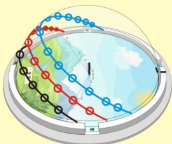
太阳轨迹 Solar trajectory
