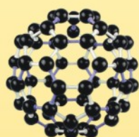
碳60模型 Carbon-60 model
