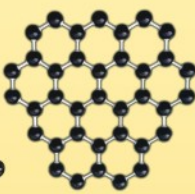
石墨烯模型 Graphene model
