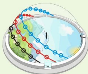
太阳轨迹 Solar trajectory
